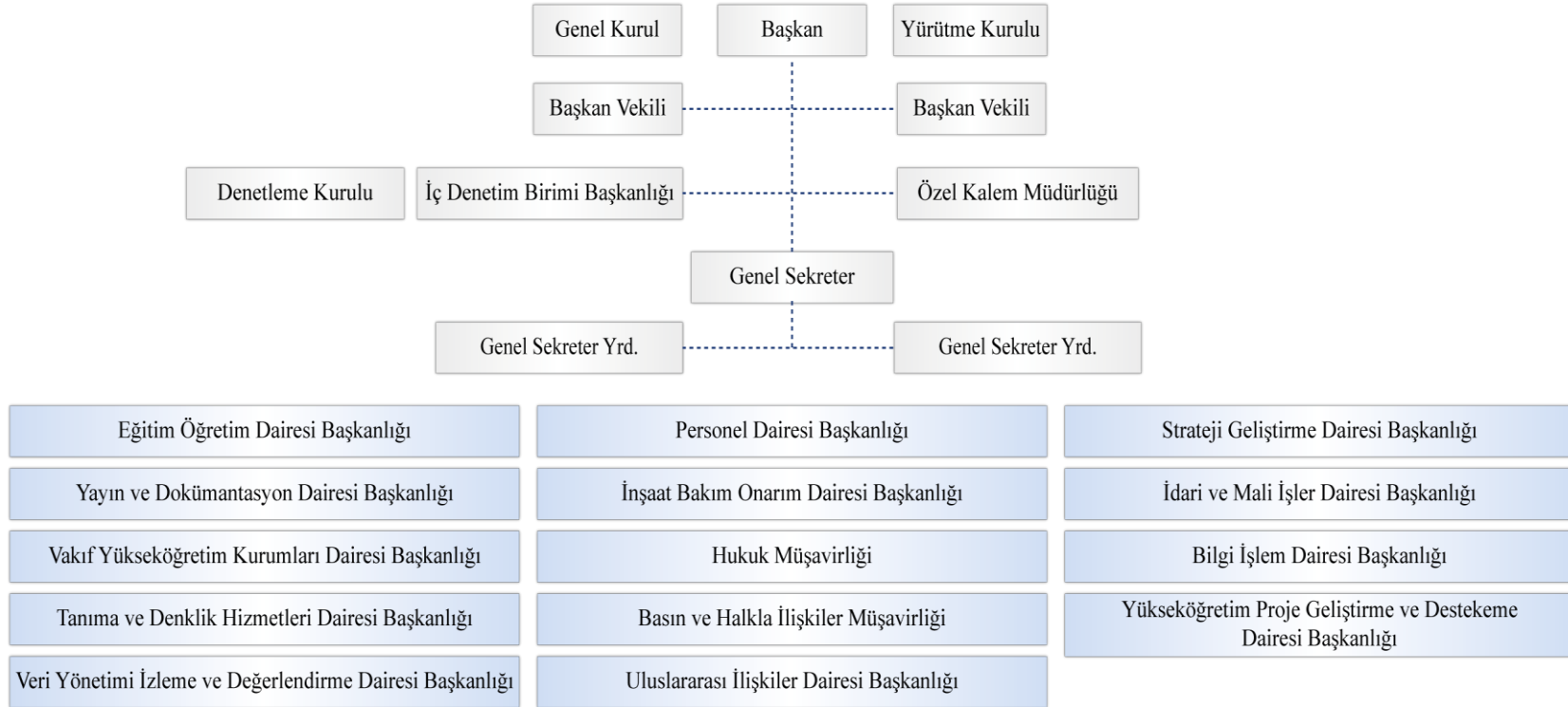
Şekil 1 Teşkilat Şeması
